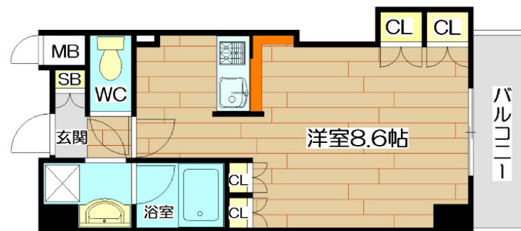
【間取り図】
