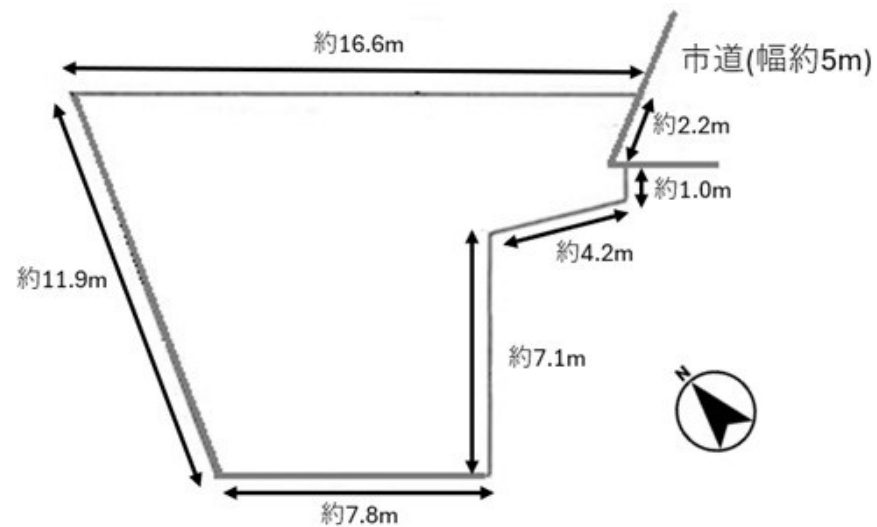
【区画図】
